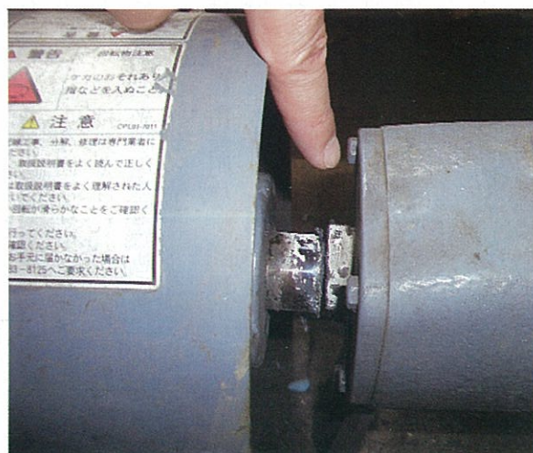
地盤沈下によるポンプシャフトの破断
